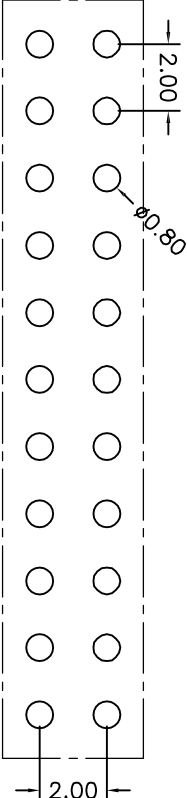
P.C.B LAYOUT
