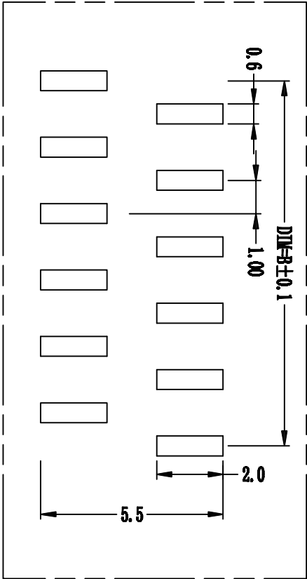
PCB Layout 正脚
